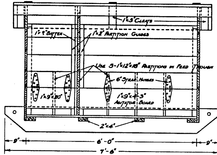
LONGITUDINAL SECTION
