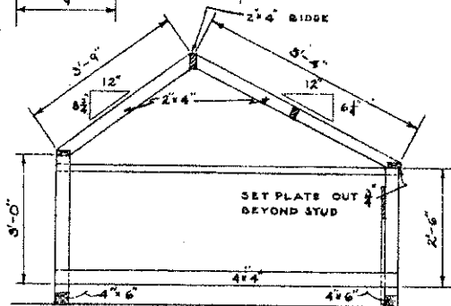
END ELEVATION
