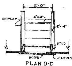
PLAN D-D
