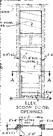
PLAN A-A
