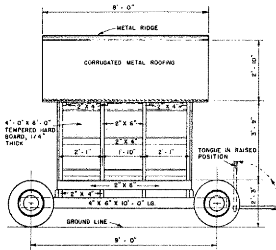
ELEVATION SCALE: 0 1 2 3 FT.
