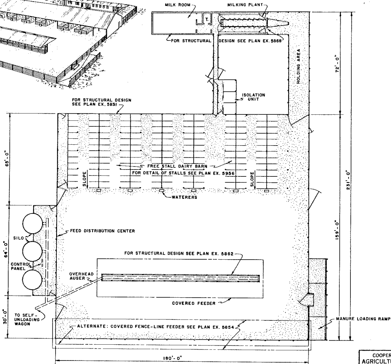
PLAN SCALE: 0 10 20 30 FT
