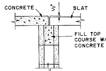
DETAIL I-A
