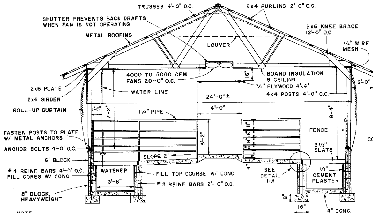
SECTION A-A
