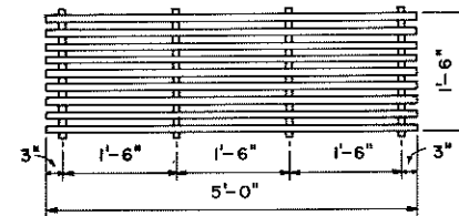
SLAT DETAIL SCALE: NONE
