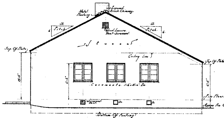
SIDE ELEVATION Scale: 1/4" = 1'-0"
