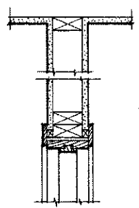
INTERIOR DOOR FRAME •
