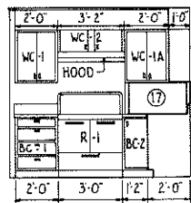
ELEVATION-A
