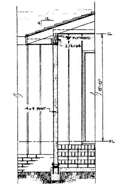
PORCH DETAIL SCALE: 1/2" = 1'-0"
