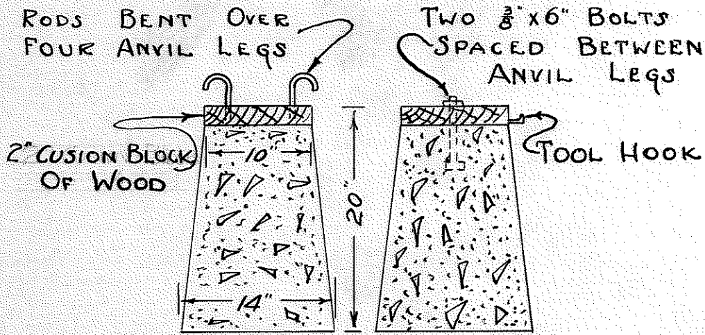
CONCRETE ANVIL BASE SCALE: 1" = 1'-0"
